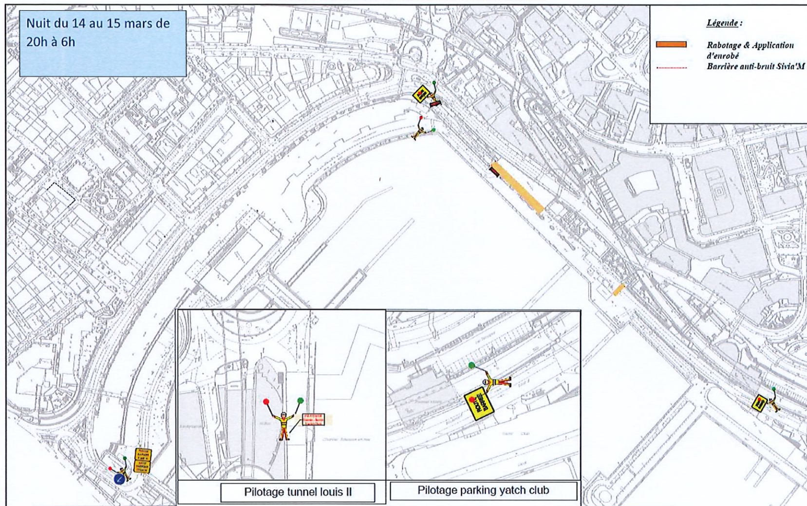
FIGURE 4 : PLAN D'INSTALLATION DE CHANTIER LUCIANA
